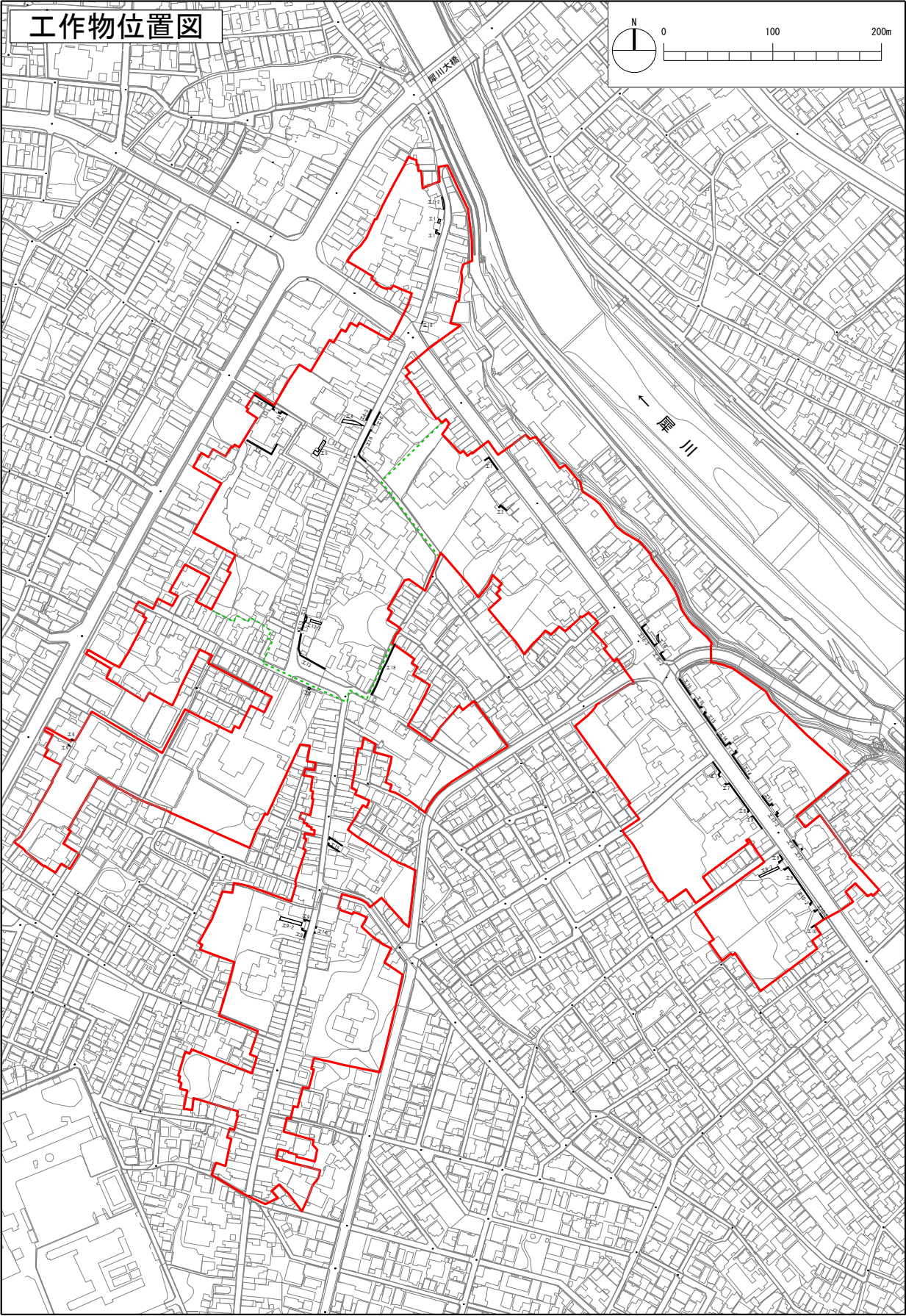
別図第 3－1 伝統的建造物（工作物）に係る図面（全体）
