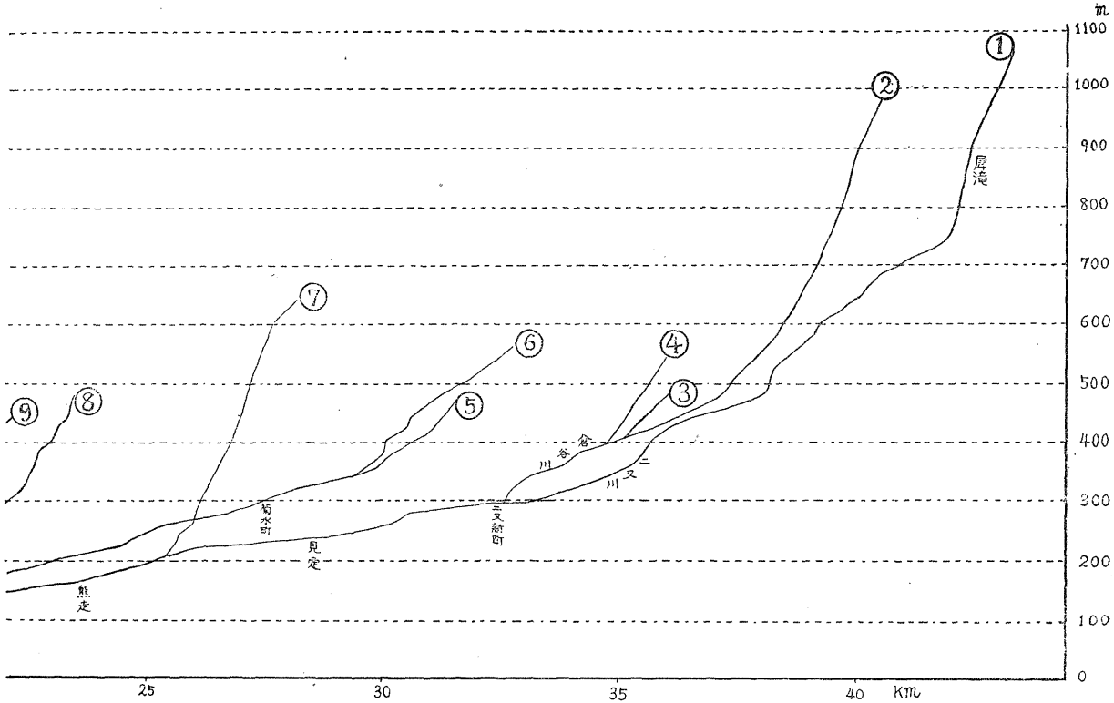
水 系 縦 断 図
