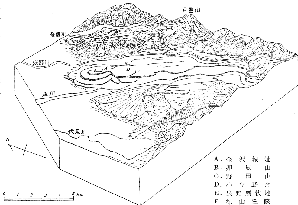
第1図 金沢市街周辺の地形
