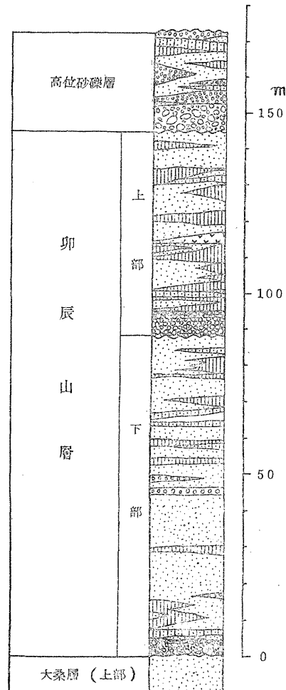
第7図 卯辰山における地層の模式柱状図。 (卯辰山の各地区における層序・層相) を総合的に表現したもの
