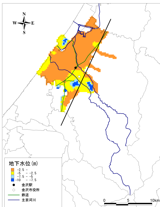
図 2-5-1 地下水位分布
