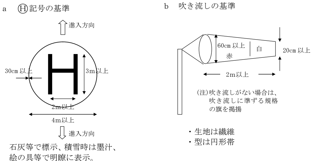
図3-10-4 H記号及び吹き流しの基準
