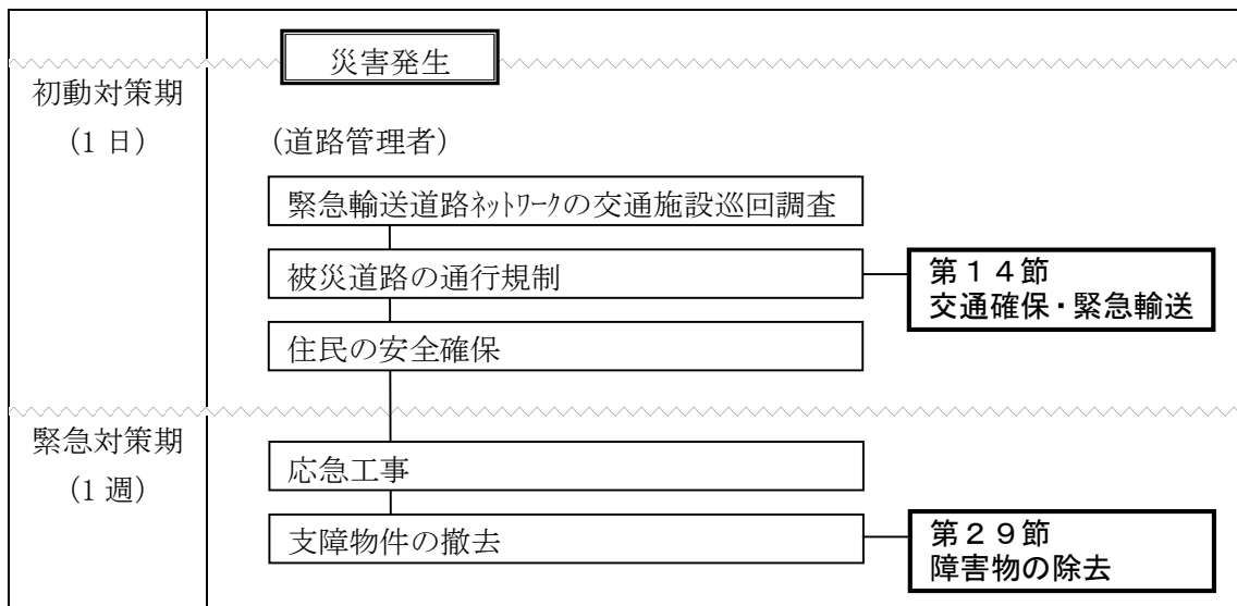
図3-28-1 道路施設の応急対策のフロー
