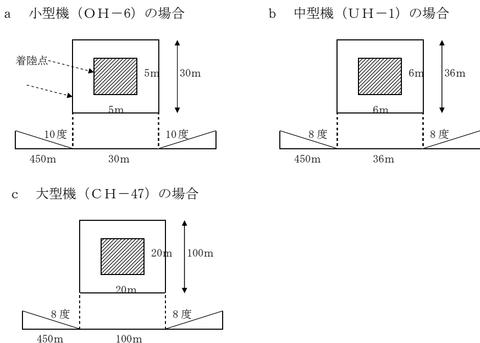
図3-10-3 ヘリコプターの機種別による着陸地点及び無障害地点の基準
