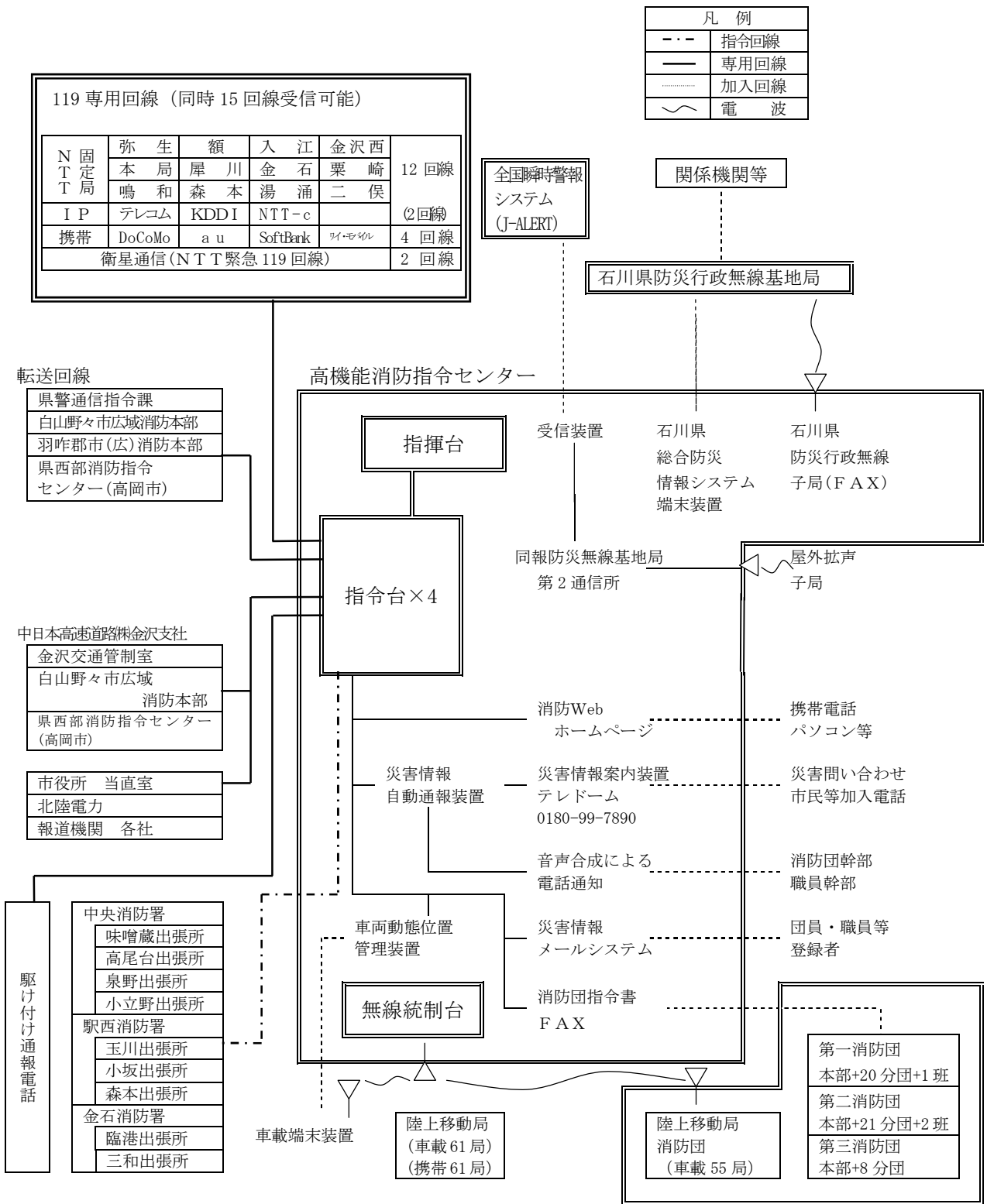
図3-9-3 消防通信系統
